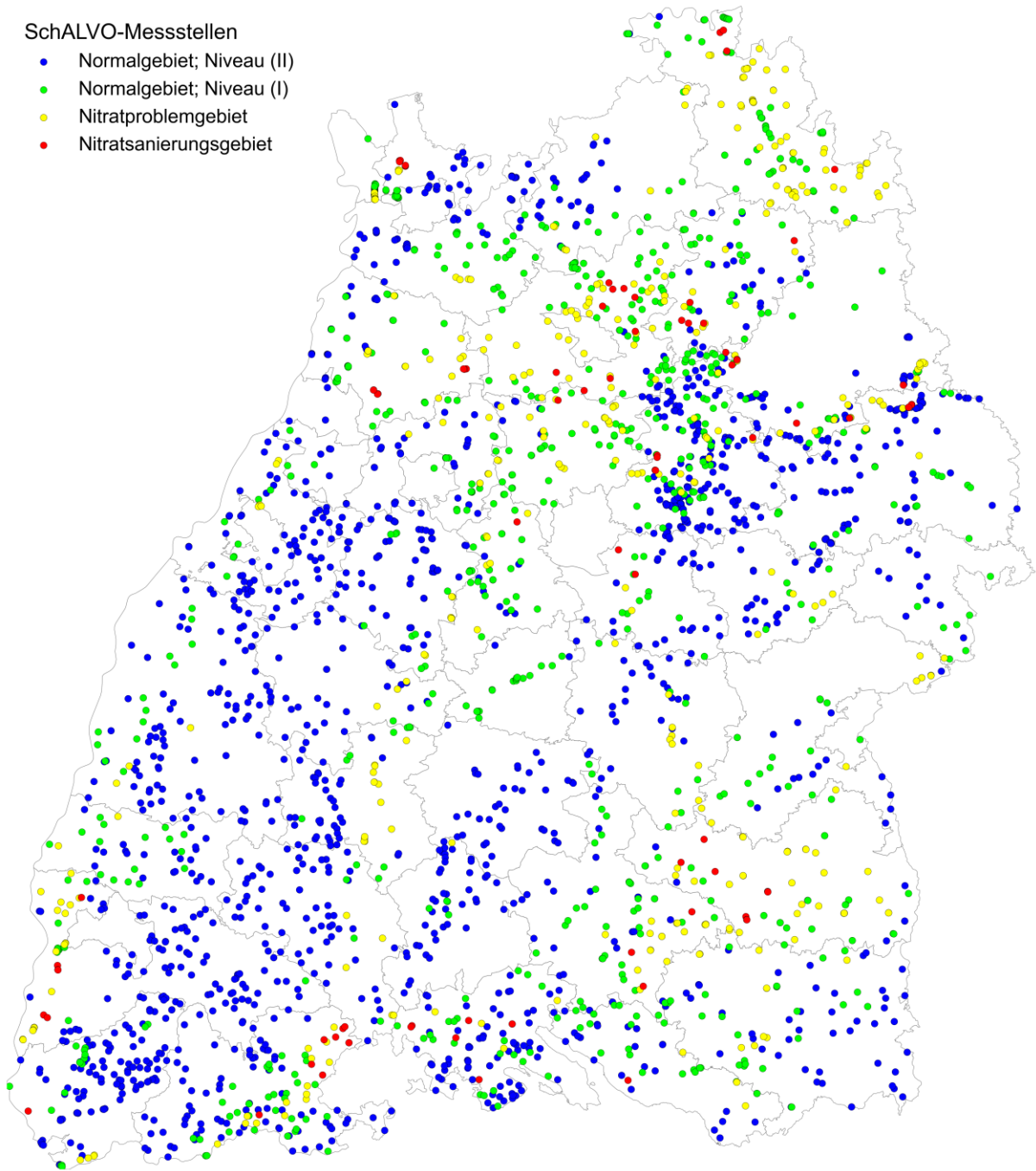
Abb. 2: Regionale Verteilung der SchALVO-relevanten Messstellen (2.718 Messstellen) mit Klassifizierung nach Normal-, Problem- und Sanierungsgebiet
